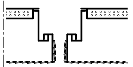
Rahmen innenliegend
