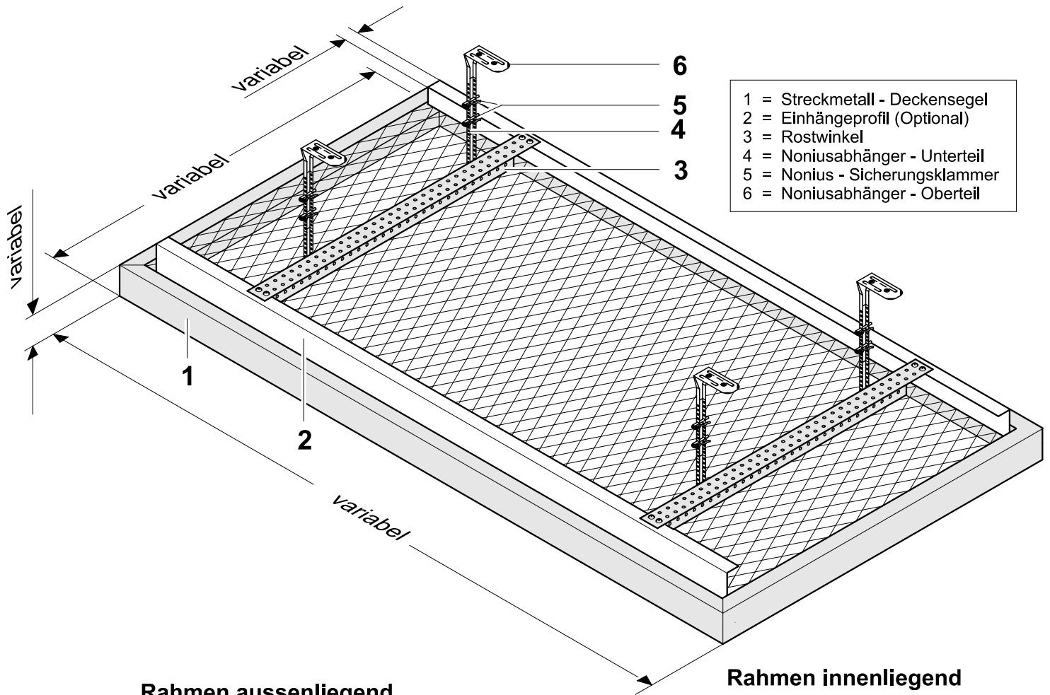
Rahmen aussenliegend
